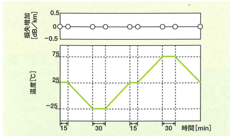
■ グラフ1 温度特性
